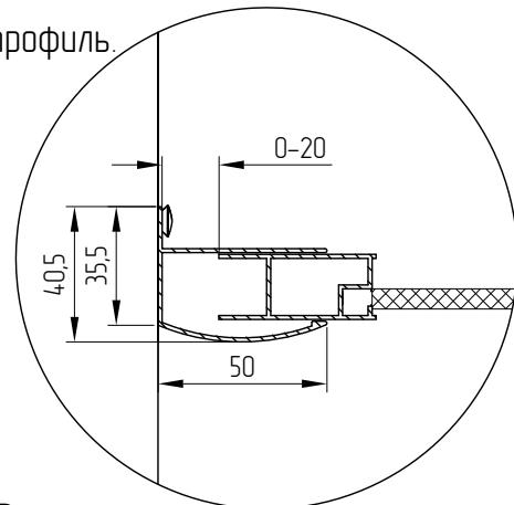
B. Соединение двери с неподвижной стенкой.
